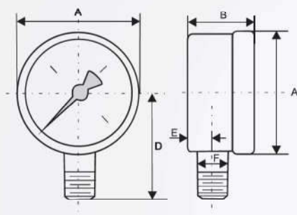
MANOMETR 100 1/4" RADIALNY
