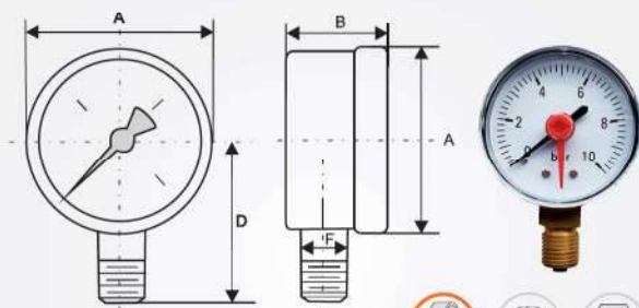
MANOMETR 50 1/4" RADIALNY
