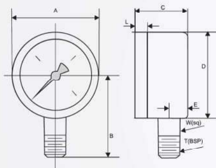
MANOMETR 63 1/4" RADIALNY
