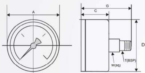
MANOMETR 63 1/4" AXIALNY
