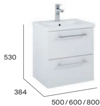
Szafka łazienkowa Compacto (do kompletacji z umywalką)
